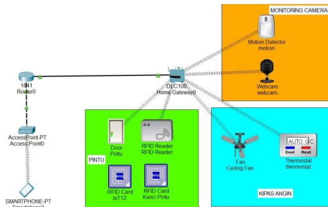
Gambar 2. Rancangan Topologi
